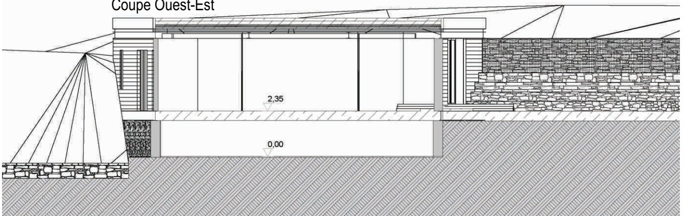
Coupe Ouest-Est
