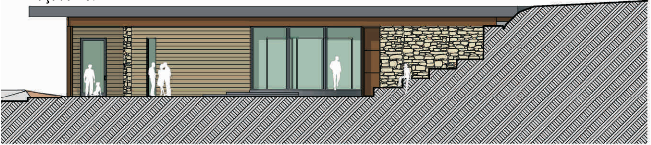
Façade Est
